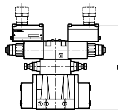
DSP*K*-/D
