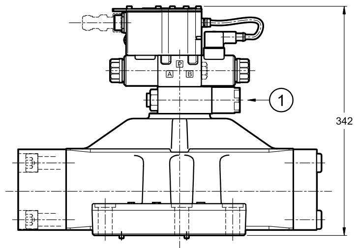
DSPE10G
