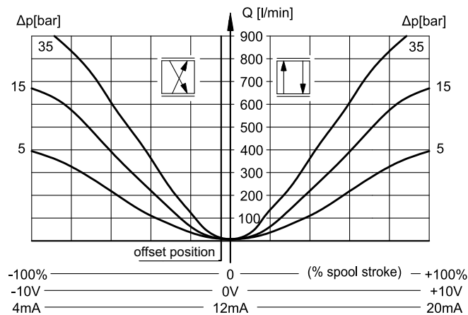
SPOOL Z400
