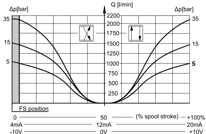
SPOOL Z1000TB
