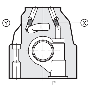
DXRE7J
