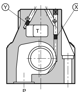
DXRE8J
