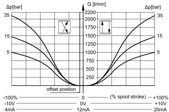
SPOOL Z1000
