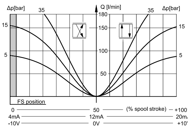
SPOOL Z100TB
