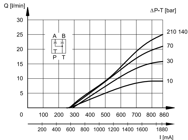
SPOOL TYPE A08
