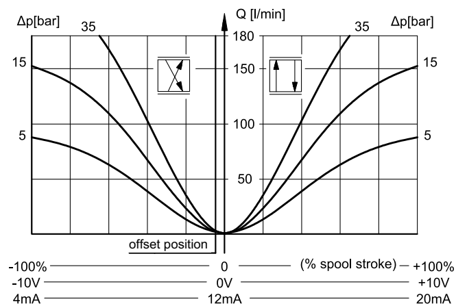
SPOOL Z100
