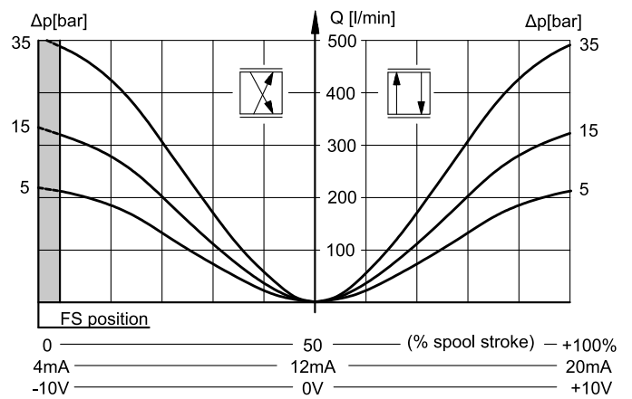
SPOOL Z220TB
