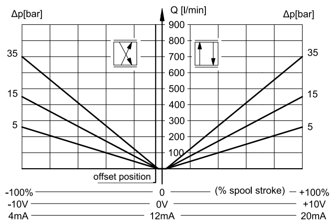
SPOOL Z250
