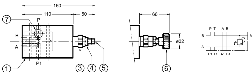
RPC1-K/M/PCT3
