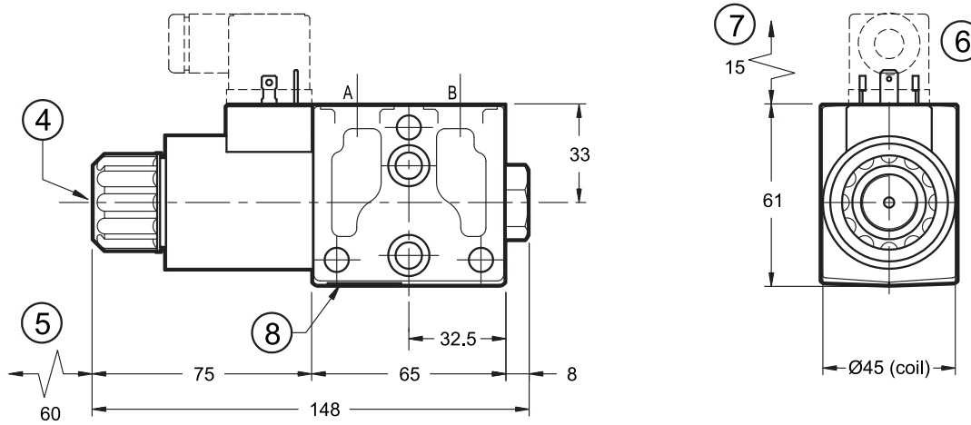
BDS3-B38
