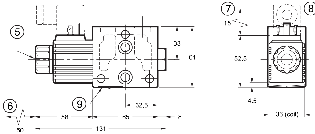
BDL2-B38
