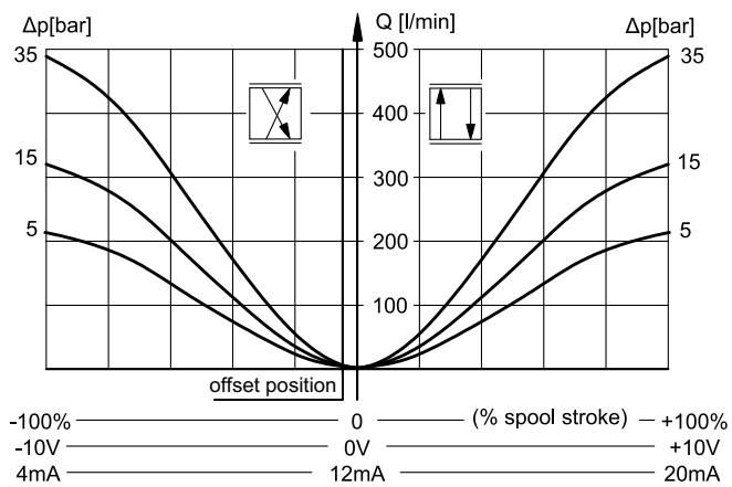
SPOOL Z220
