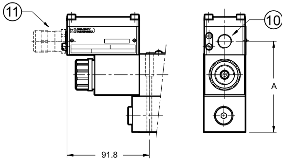
PRE3K*-/10*-*K9S*
