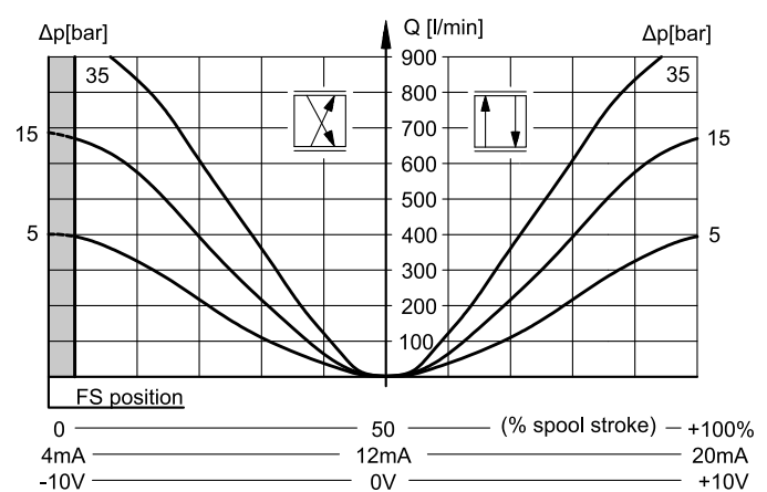
SPOOL Z400TB
