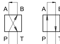
SPOOL TYPE A08
