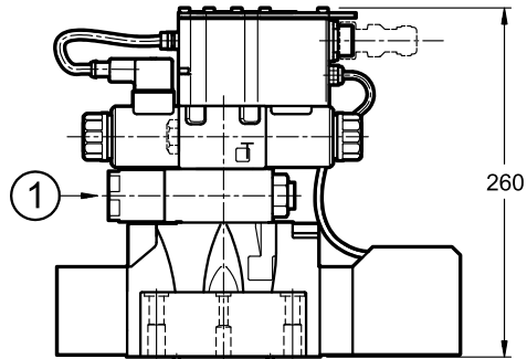
DSPE7J
