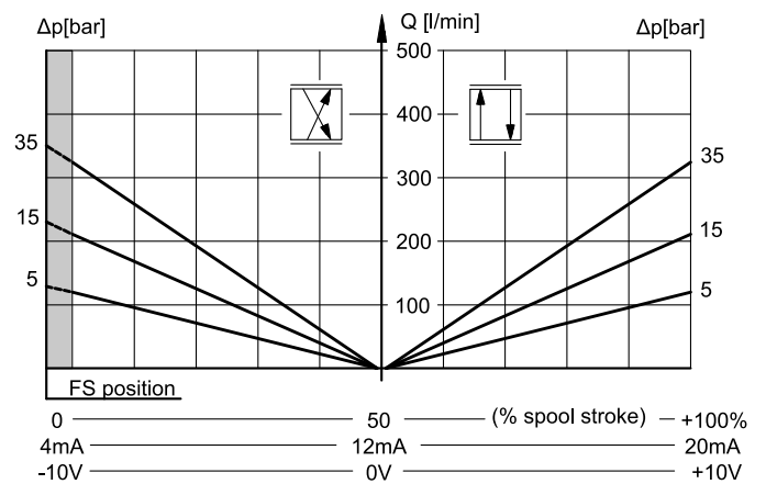
SPOOL Z120TB
