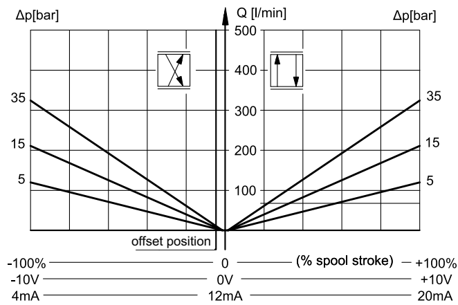
SPOOL Z120
