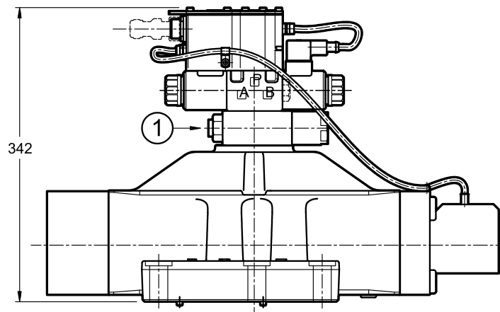
DSPE10J / DSPE11J
