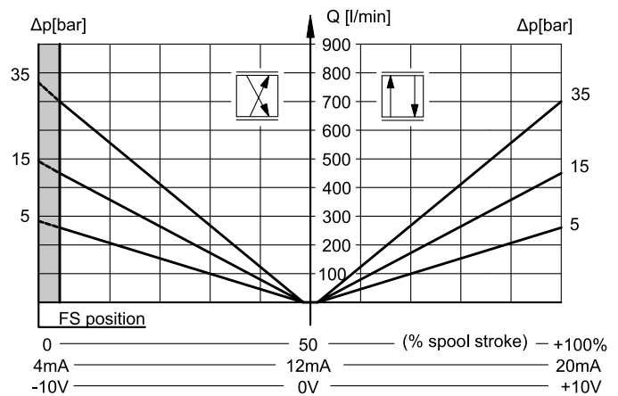
SPOOL Z250TB
