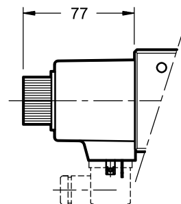
MDS5-*/10*-A*
